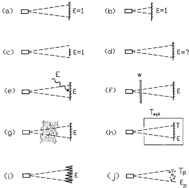
Figur 4. (a) simpel pyromettermåling på emne med emissionskoefficient på 1, (b) afstanden til emnet har normalt ingen betydning såfremt emnet er indenfor synsfeltet, (c) udfylder emnet ikke synsfeltet vil der kunne begås store målefejl, (d) normalt er emissionskoefficienten ikke kendt for overfladen, (e) refleksion af stråling fra andre varmere flader kan give betydelige målefejl, (f) et målevindue kan påvirke målingen kraftigt, (g) atmosfæren/mediet som der måles igennem kan absorbere eller emitte stråling og give anledning til målefejl, (h) det kan være vanskeligt at måle temperatur på emner i en varm ovn, (i) en overflades effektive emissionskoefficient øges med øget overfladeruhed (f.eks. gevind eller slibning) og (j) måling af overfladetemperatur af gasbårne partikler eller gastemperatur (f.eks. kulstøv forbrænding).
